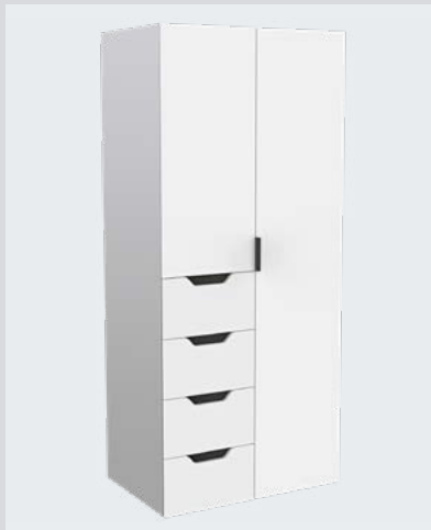
2048H x 900W x 580D 1x Cabinet Shell I/N: 0430513 4x Scallop Drawers I/N: 0430661 1x Door Right I/N: 0430792 1x Door Left I/N: 0430754 3x Hinge 110 I/N: 0431437
