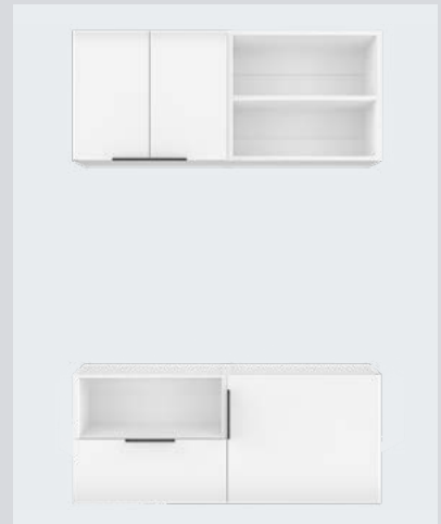
2 x 512H x 1200W x 380D 4x Cabinet Shell I/N: 0431420 2x Adj Shelves 2pk I/N: 0430838 1x Dbl Doors I/N: 0430549 1x Door Right I/N: 0431283 1x External Drawer I/N: 0430710 3x Hinge 110 I/N: 0431437
